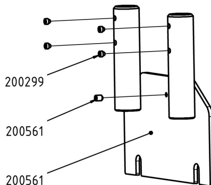
Detail Stabverschraubung
