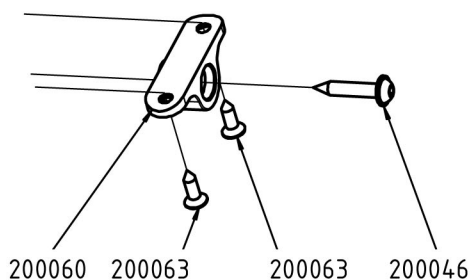
Detail Handlaufverbinder
