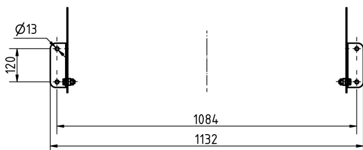
Bohrbild Fußwinkel A-A
