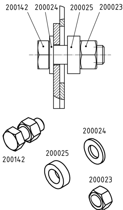
Detail Verschraubung
