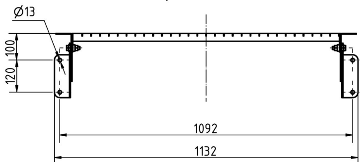
Maße für Stufenbreite 100 cm Bohrbild Kopfwinkel B-B
